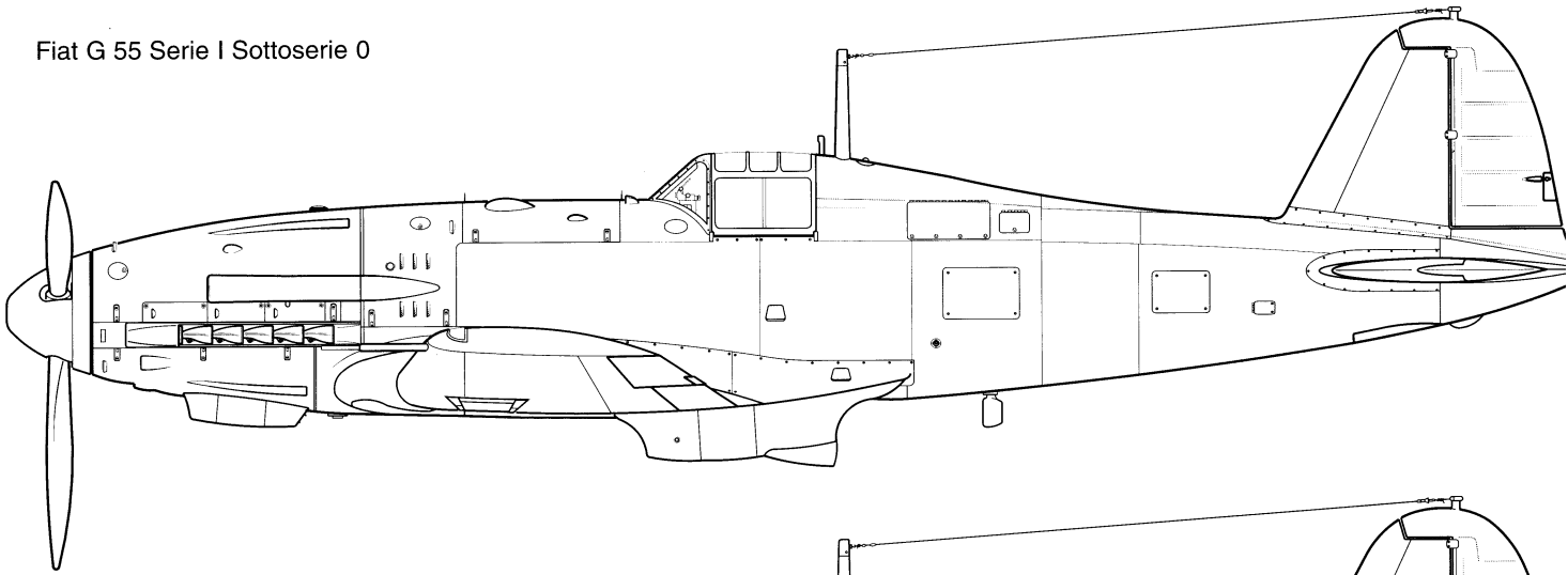
Fiat G 55 silurante
