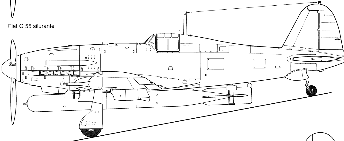
Fiat G 55 B
